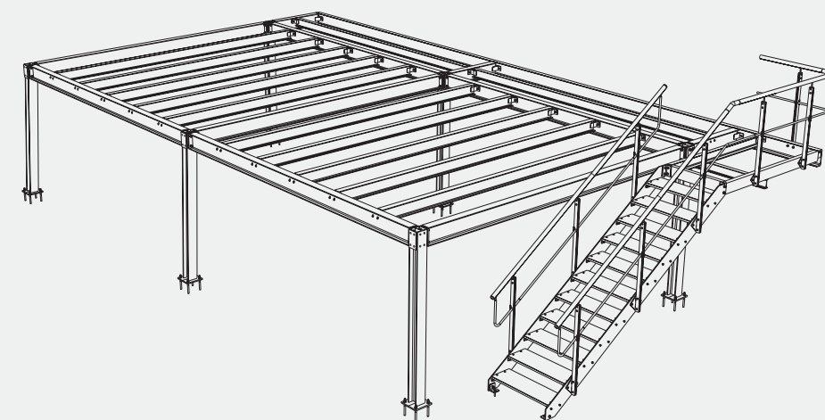
Stand sicher ohne störende Diagonalverstreben: die Stahlbau-Bühnenkonstruktion von Nerling mit hochfest verschraubten Knotenpunkten.
