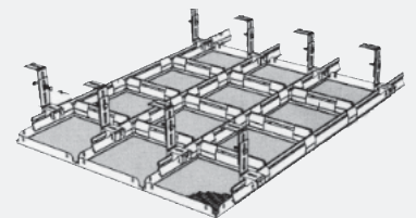
Mineralwolle-Deckenplatte Struktur „Galaxie“
